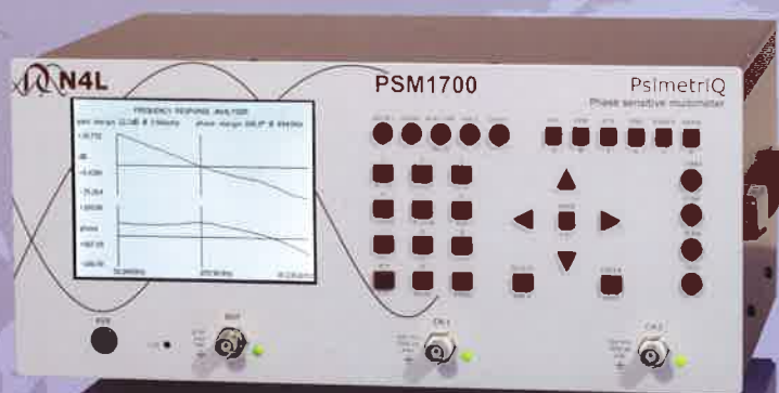
PSM1700 带宽 10uHz ~ 1MHz
