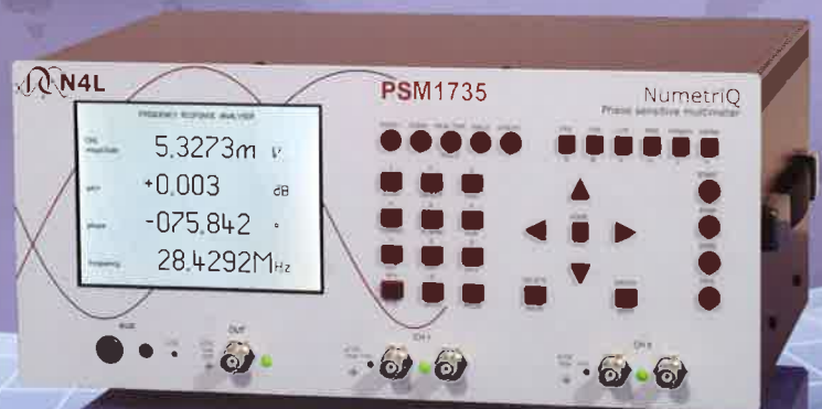
PSM1735 带宽 10uHz ~ 35MHz
