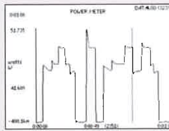
▲ 瓦特曲线及游标指出第2351记录
