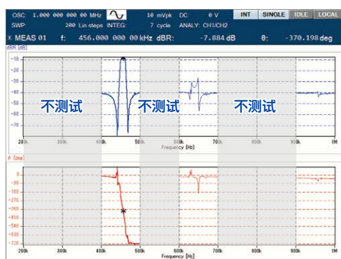
滤波器的通带测试 仅必要频率范围的测试
